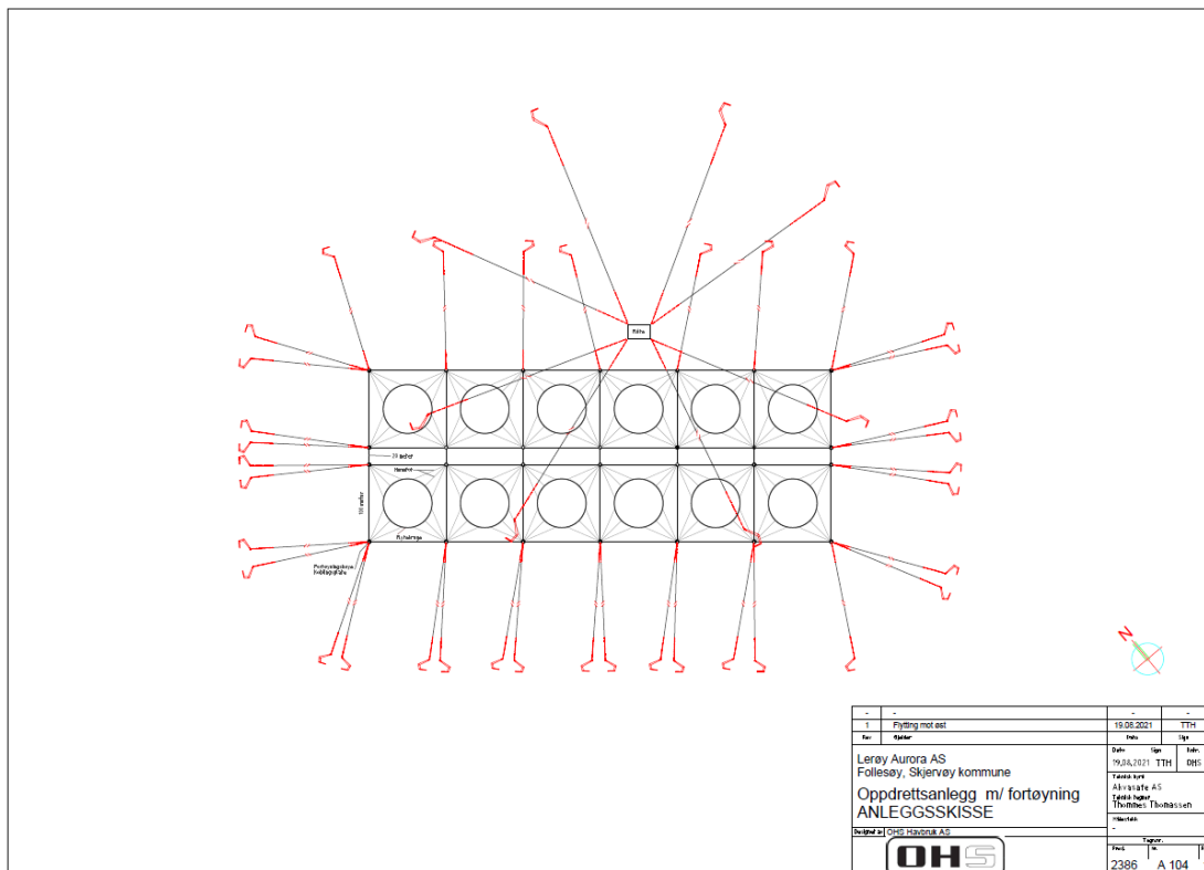
Figur 5 Viser anleggsskisse. Ømsøkt anlegg består av 12 burs rammefortøyning med 20 meter bred servicekorridor og med tilhørende forflåte
